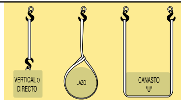
Eslingas Planas
