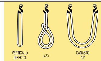
Eslingas Circulares
